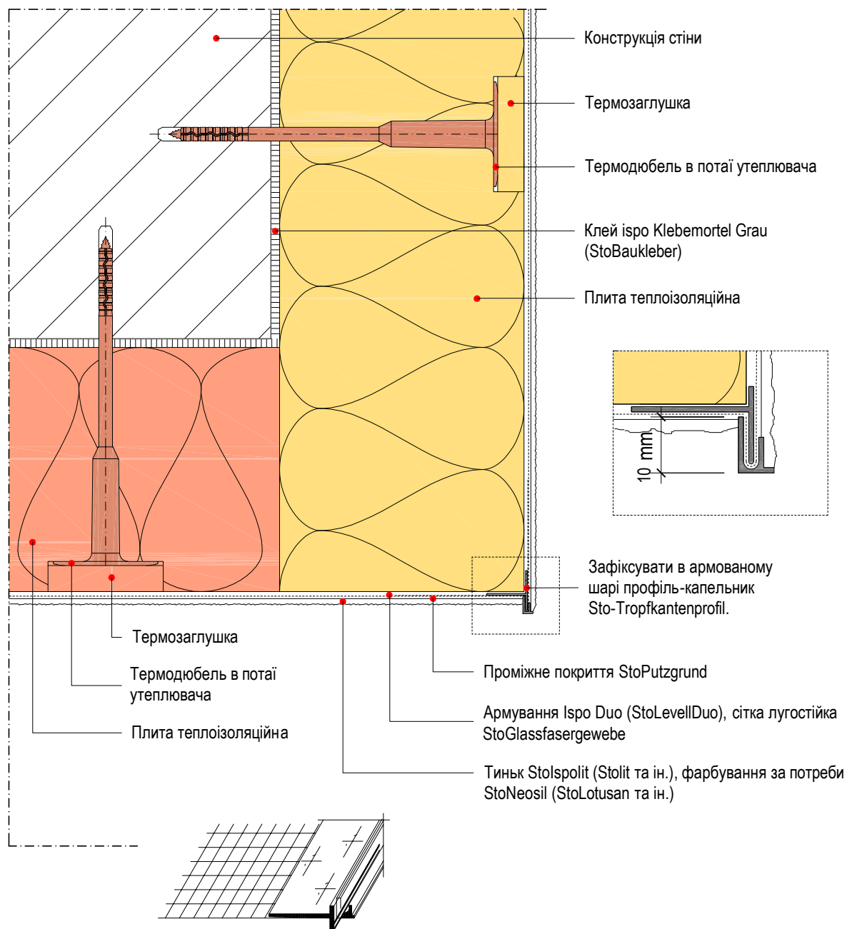
З'єднання профілю Sto-Tropfkanten з'єднувачем
